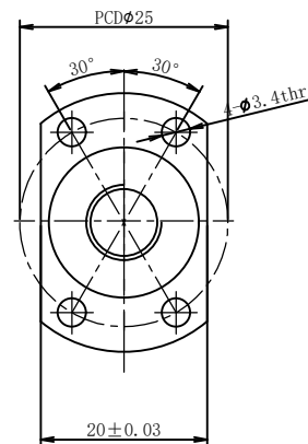
滑块尺寸
