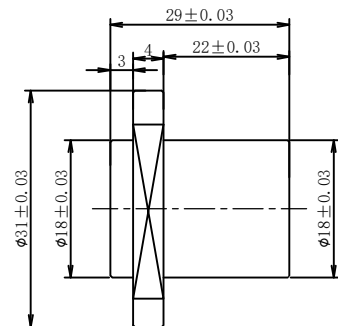
滑块尺寸
