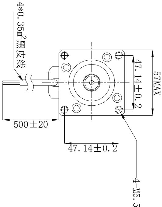
接线图/Wiring Diagram
