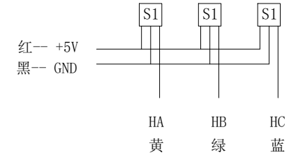
霍尔接线图
