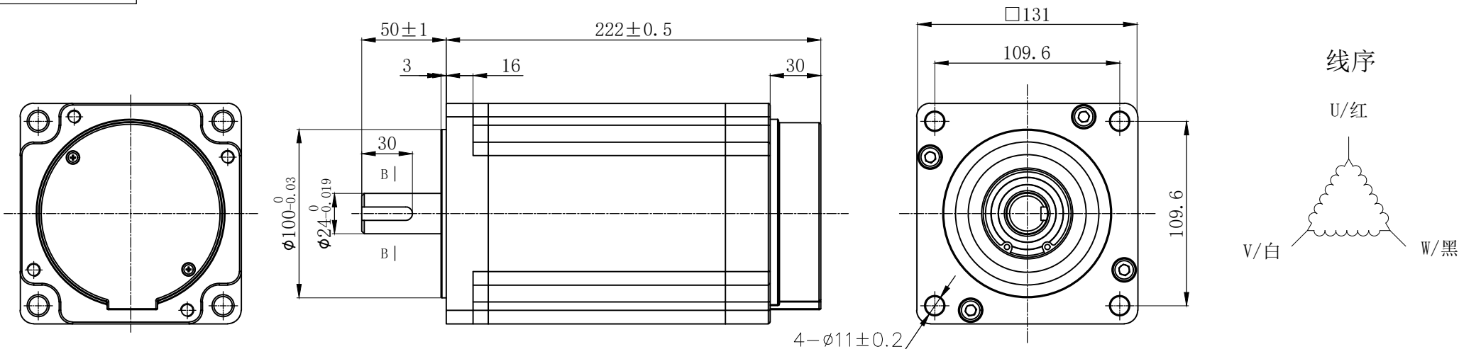
接线图
