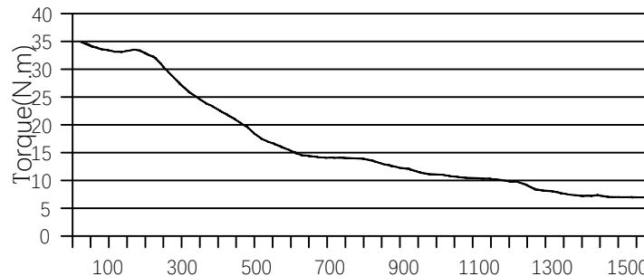
动态力矩曲线
