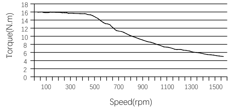
动态力矩曲线
