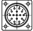
绝对式编码器连接器
