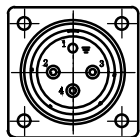
增量式编码器连接器
