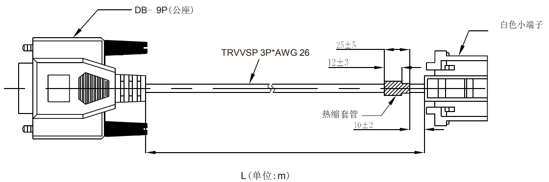
编码器接线
