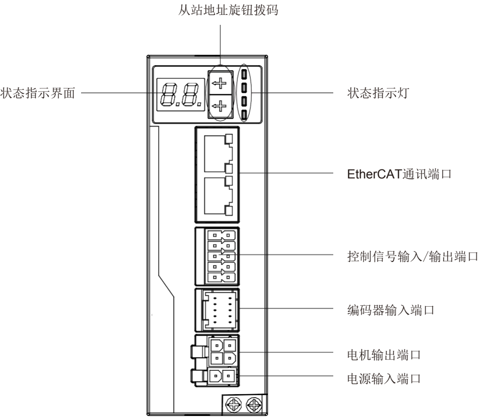
驱动器侧面端口示意图
