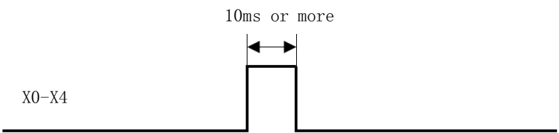
X0-X4 时序图
