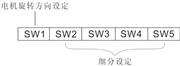
拨码开关组合图
