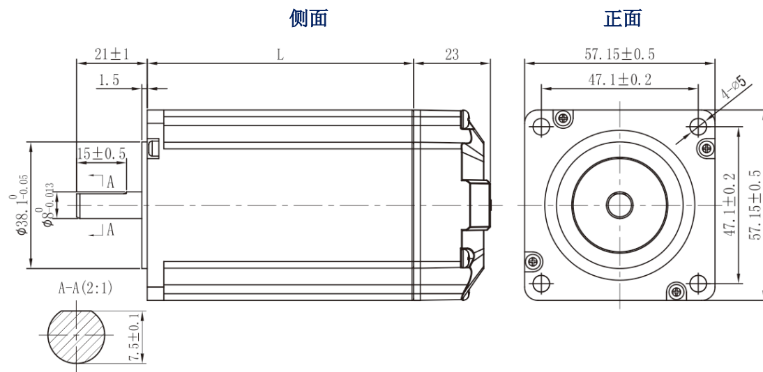
安装尺寸图 (单位: mm)
