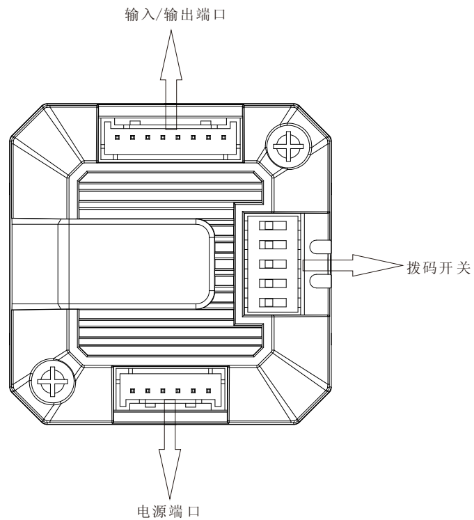
驱动器接线示意图
