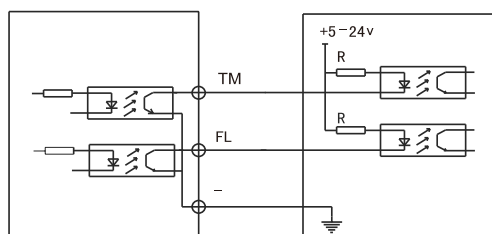
驱动器
