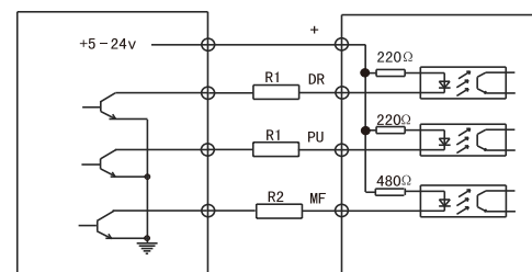
控制器
