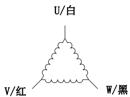
接线图/Wiring Diagram
