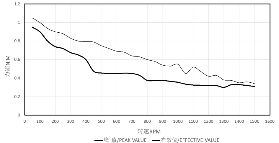
力矩曲线
