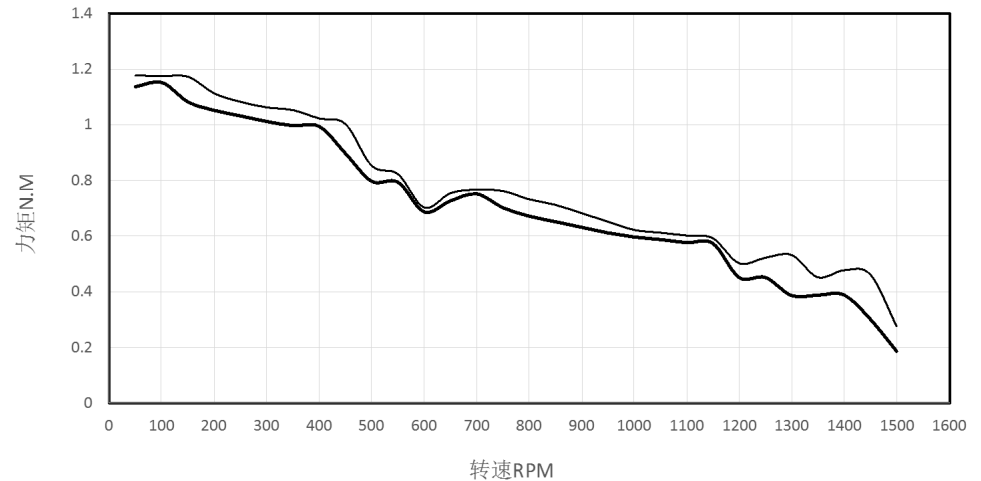
力矩曲线
