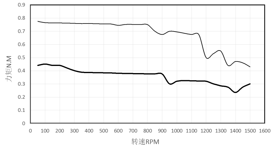
力矩曲线
