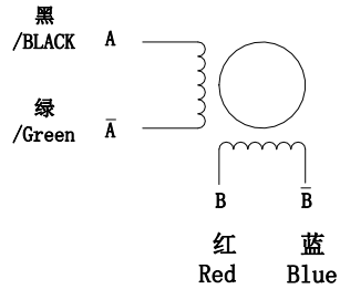
Wiring Diagram/接线图
